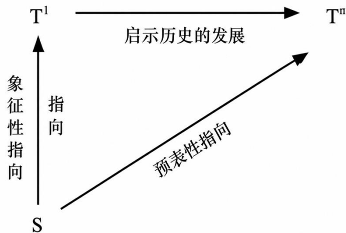
图 6.1：克劳尼三角结构
